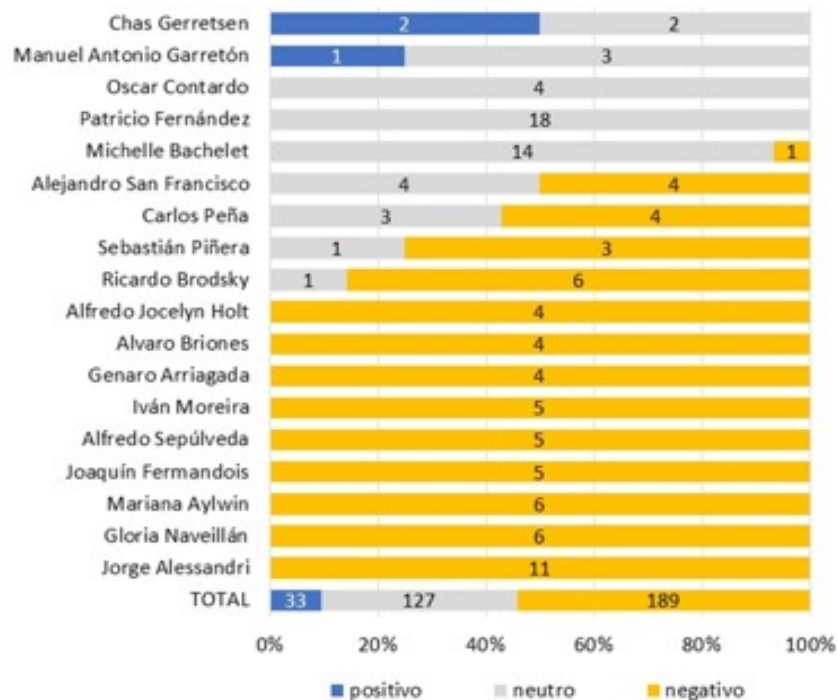
Gráfico 19. Opiniones de actores sobre LA UNIDAD POPULAR
