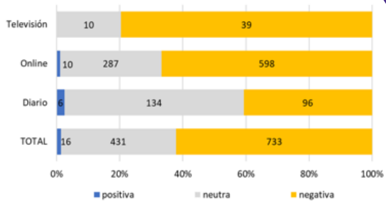
Gráfico 13. Valoración EL GOLPE MILITAR / LA DICTADURA en artículos de prensa según tipo de medio
